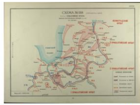
Рижская операция 1944 г.
