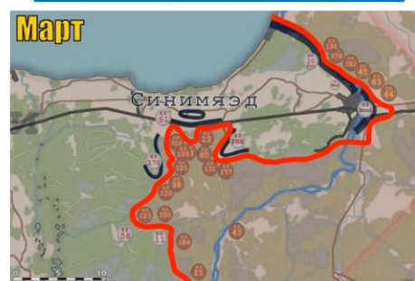
Положение РККА в ходе Нарвской операции в марте 1944 г.
