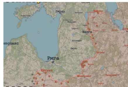
Положение Красной Армии перед началом Прибалтийской операции, сентябрь 1944 г.
