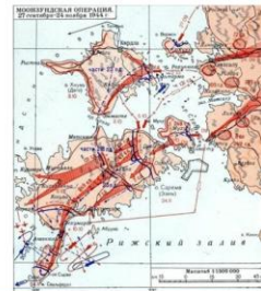
Моонзундская операция 1944 г.
