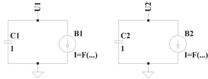
Рисунок 1 - Концепция построения схемотехнических аналогов биологических нейронов. Пример на рисунке соответствует модели второго порядка в виде системы уравнений
