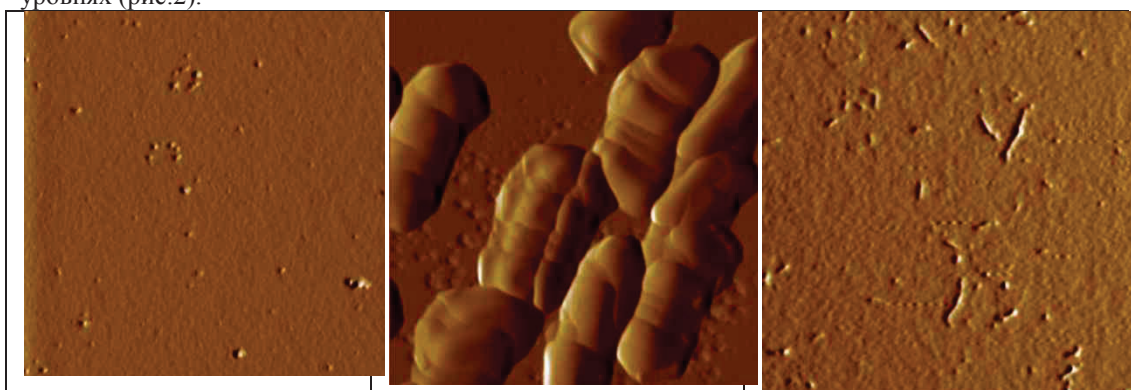
Рис. 2. АСМ - изображение, размер 3х3 мкм: а - 10% САЧ; б - 10%+6% NaCl; в - 10%+8% NaCl Определение параметров микрорельефа пленок показало, что на микроуровне шероховатость поверхности пленки САЧ увеличиваются с повышением концентрации соли в растворе по линейному закону (рис.3а), что хорошо согласуется с изменением морфологии пленки. Для растворов 10% САЧ с добавкой соли характерны крупные удлиненные агрегаты типа пластинчатых и фибриллярных структур вместо тонкодисперсной сетчатой структуры (рис.2б,в).
