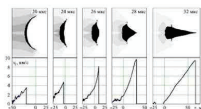
Рис. 3. Формирование кумулятивной струи зарядом с полусферической облицовкой дегрессивной толщины 2.4 мм/1.0 мм.
