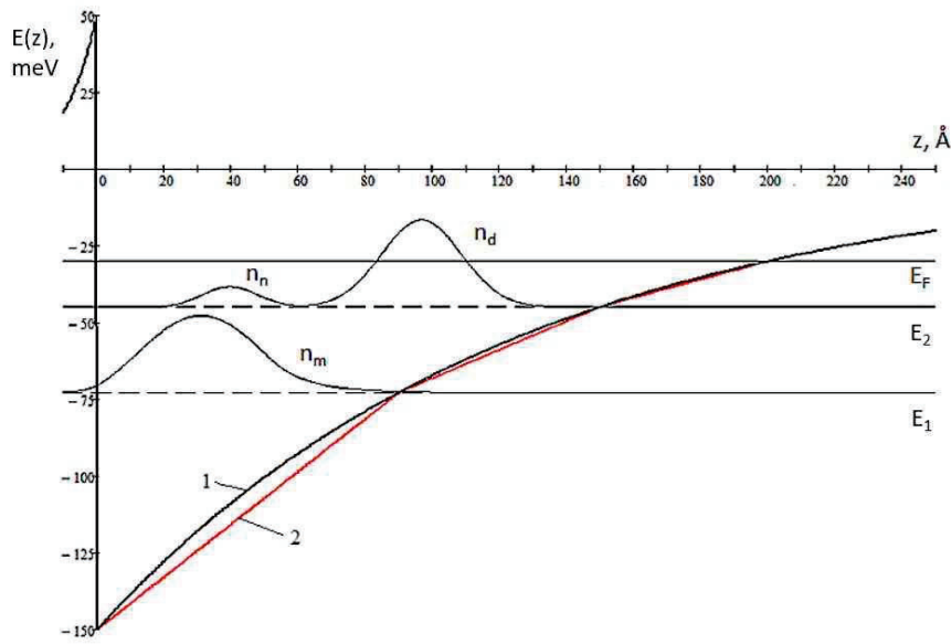
Рис. 1. Энергетическая диаграмма зоны проводимости E_c(z) гетероперехода с двумя заполненными подзонами размерного квантования E_1 и E_2 ; n_m и n_{n,d} – поверхностные концентрации 2D электронов, E_F – энергия Ферми.
