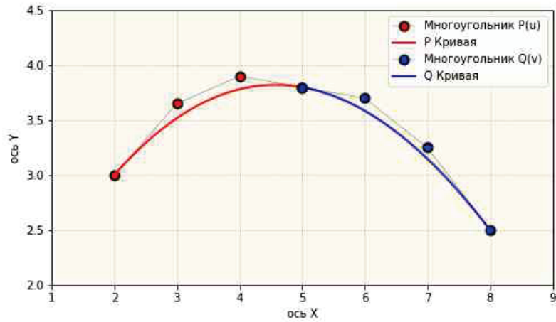
Рис.2. Пример гладко сопряженных кривых Безье
