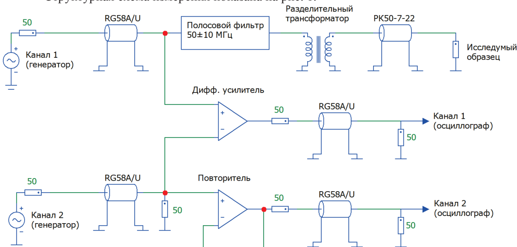
Рис. 1. Высокочастотная схема измерения проводимости.
