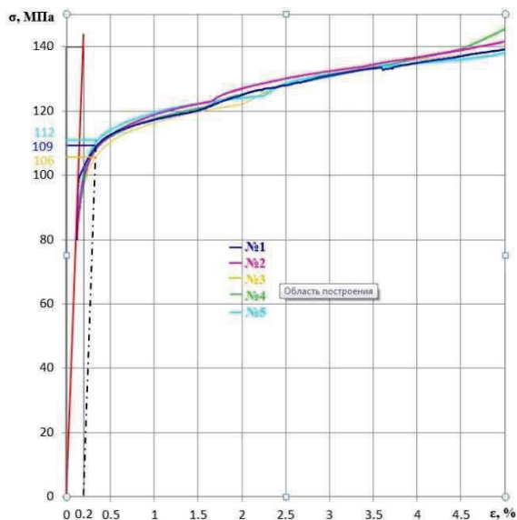
Рисунок 3 – Диаграммы деформирования при сжатии пятикратных образцов из сплава АМцС
