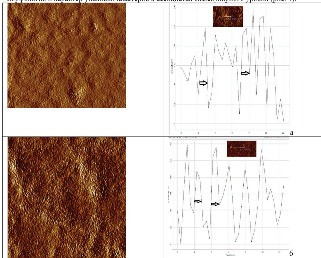
Рис.4- АСМ - изображение белковой сети с профилем сечения, скан 100х100нм: а - 10%САЧ; б- 10%САЧ+6%NaCl. Стрелки показывают размер первичной глобулы порядка 1-2нм.
