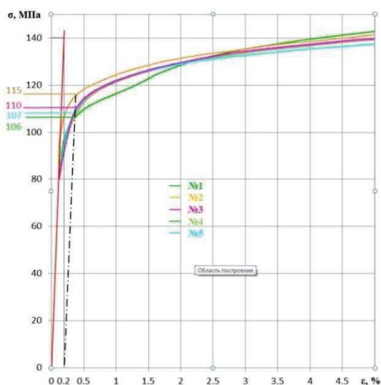
Рисунок 2 – Диаграммы деформирования при сжатии двукратных образцов из сплава АМцС
