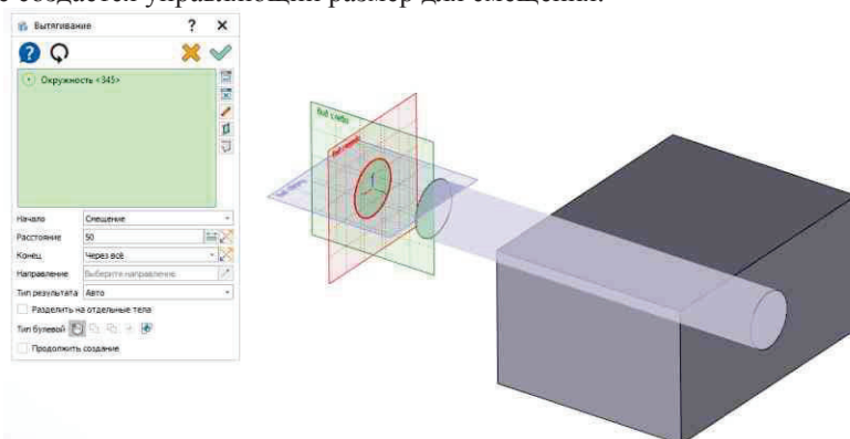
Рис. 5. Вытягивание со смещением, равным 50 и режим конца вытягивания через всё На рисунке 6 изображён пример вытягивания со смещением через всё с применением булевой операции вычитания на единственный твердотельный объект на сцене.
