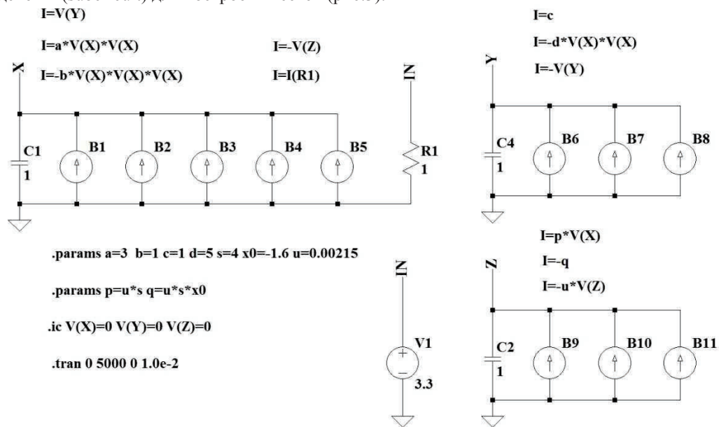
Рисунок 2 - Идеализированная радиотехническая модель ХР биологического нейрона
