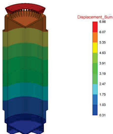
Рисунок 3 – Результирующие перемещения U_{Sum} конструкции ТУК, мм
