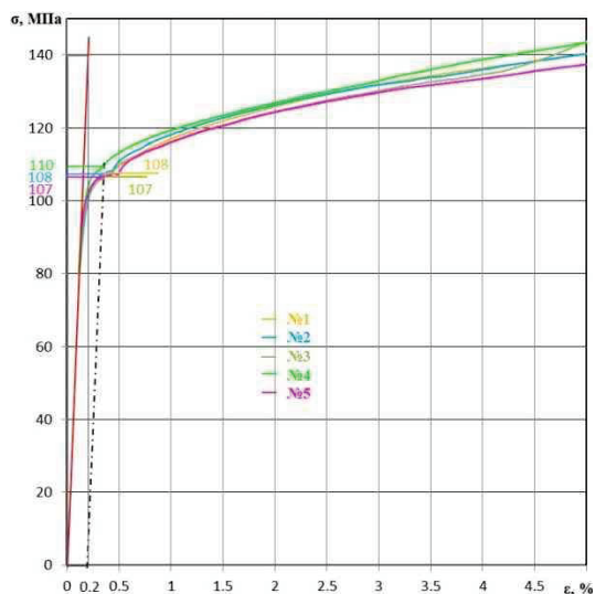
Рисунок 5 – Диаграммы деформирования при сжатии десятикратных образцов из сплава АМцС
