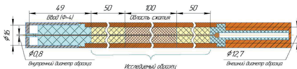
Рис. 2. Упрощенная геометрия коаксиальной камеры сжатия для исследуемого образца.
