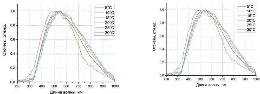
Рисунок 2 - Спектры СЛ в системе дистиллированная вода – воздух и формамид – воздух при температуре 5 – 30 °С
