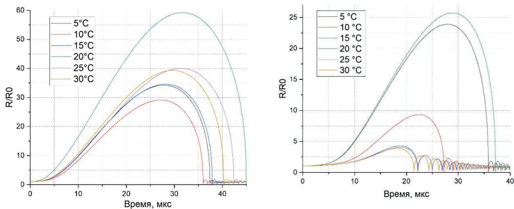
Рисунок 1 - График зависимости \frac{R(t)}{R_0} в диапазоне температур от 5 °С до 30 °С для системы формамид - воздух и вода - воздух
