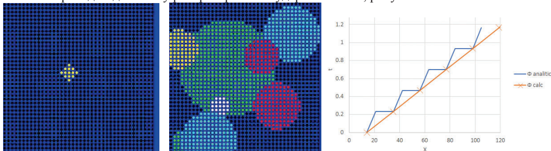
Рисунок 2 – Динамика распространения ударной волны и график фронта ударной волны
