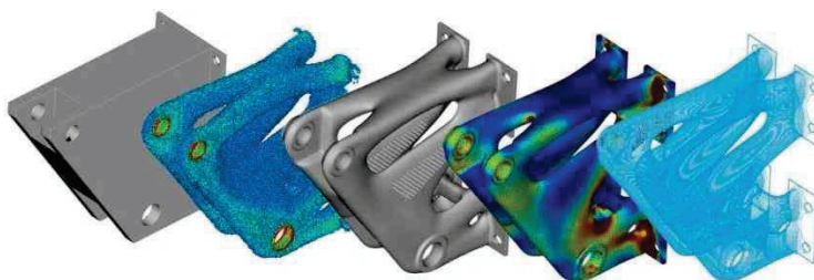
Рис. 3 – Распределение напряжений в оптимизированной конструкции
