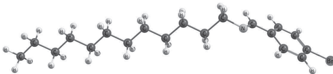
Рис. 2. Оптимизированная структура парабромпроизводного азометина с додецильным заместителем в октаноле.
