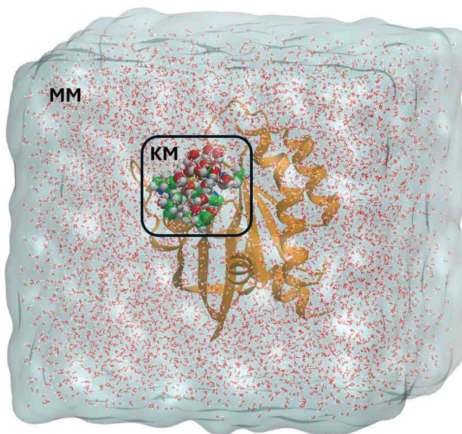
Рисунок 1. Полноатомная модель белкового комплекса KRAS с лигандом. В квантовую подсистему (КМ) включены непосредственные участники химической реакции, а также их ближайшее окружение (выделены ван-дер-Ваальсовыми сферами), прочие атомы включены в молекулярно-механическую подсистему (ММ). Цветовая схема: зеленым обозначены атомы углерода, красным – кислорода, синим – азота, белым – водорода.
