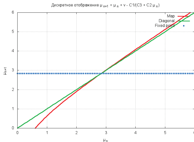
Рисунок 4 – Неподвижная точка отображения (4), соответствующая стационарному решению
