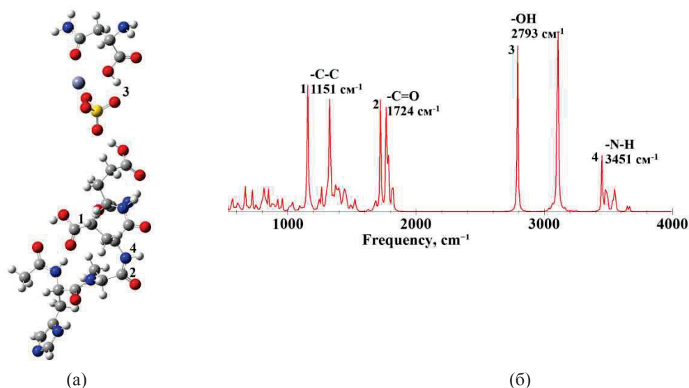
Рис. 2. Рассчитанные структуры (а) и ИК спектры (б) молекулярных комплексов молекулярных комплексов тетрапептида НАЕЕ с серином (I), глутамином (II) и аспарагином (III).
