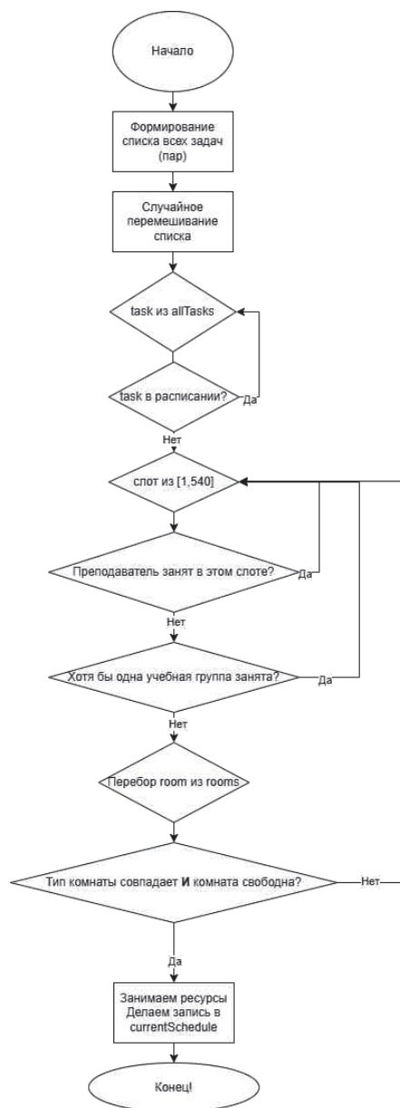
Рисунок 3. Приоритетный алгоритм
