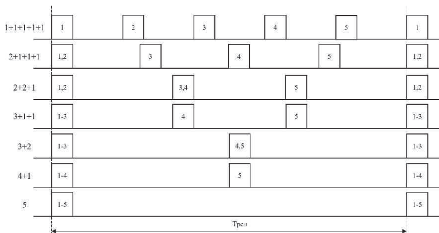
Рисунок 1 – Регулярные режимы колебаний системы из пяти нейронов
