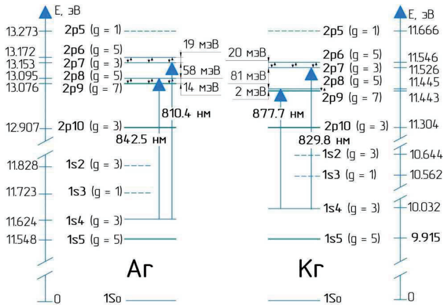
Рис. 1. Схема уровней атомов аргона и криптона с дополнительной оптической накачкой
