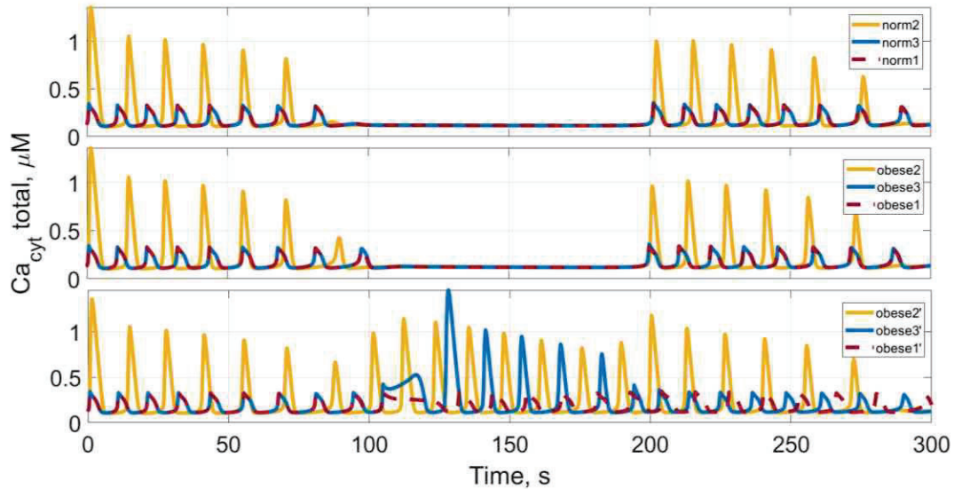
Рис. 3. Графики зависимостей средней по пространству концентрации Ca^{2+} в цитозоле от времени при двух однократных стимулах IP_3 в моменты времени 0 с и 200 с.
