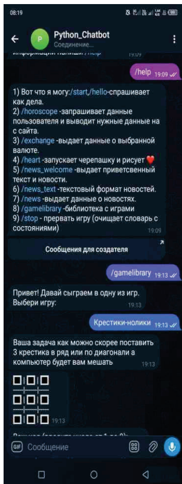
Рис. 1-интерфейс чат-бота
