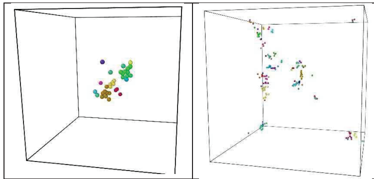
Рисунок 4 – Пространственное распределение кластеров дефектов после прохождения первичной выбитой частицы. Слева – при энергии 2кэВ, справа – при энергии 20кэВ. Разными цветами обозначается принадлежность дефектов к разным кластерам.
