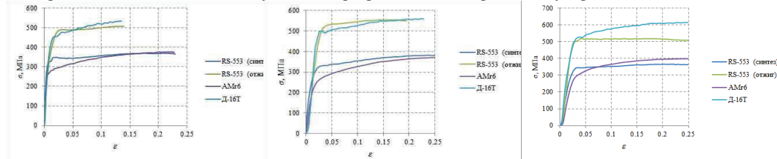
Рисунок 5 – Диаграммы деформирования алюминиевых сплавов при различных V Определённые из диаграмм деформирования значения условного предела текучести \sigma_{0,2} приведены в таблице 2.
