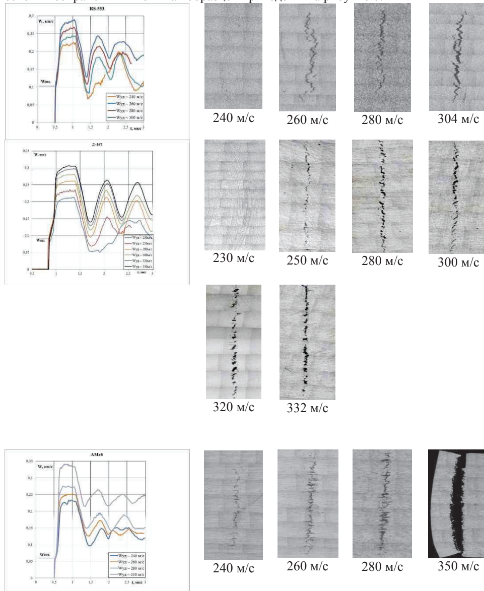
Рисунок 6 –Зависимости скорости движения свободных поверхностей образцов из сплавов RS-553, Д-16Т и АМг6. Металлография сохраненных после опытов образцов
