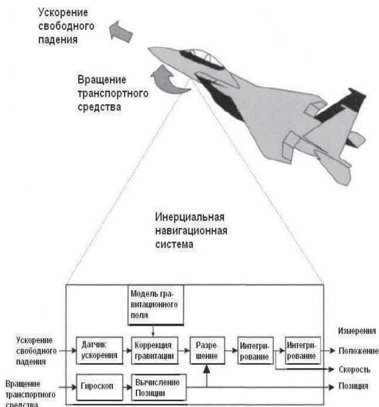
Рисунок4 – Функциональные компоненты инерциальной навигационной системы.
