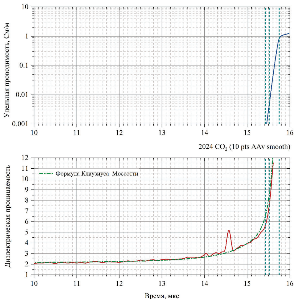
Рис. 4. Зависимость проводимости и диэлектрической проницаемости конденсированной углекислоты от времени в эксперименте с МК-1. Вертикальные пунктирные линии указывают времена срабатывания бетатронов.
