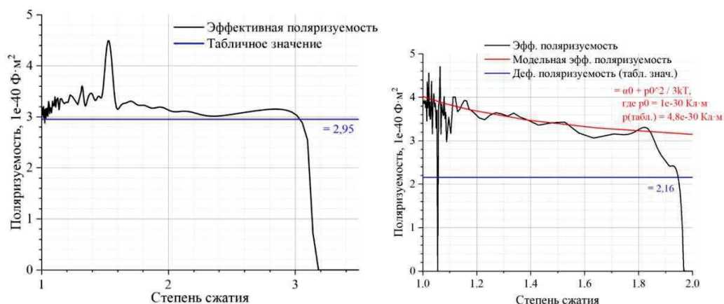
Рис. 5. Зависимости поляризуемости от степени сжатия конденсированной углекислоты (слева) и аммиака. Эффективная поляризуемость – вычисленная поляризуемость по формулам Клаузиуса-Моссотти и Дебая-Ланжевена, модельная эффективная поляризуемость – вычисленная поляризуемость, в формуле которой взято значение, в 4,8 раз превышающее табличное значение дипольного момента отдельной молекулы аммиака.
