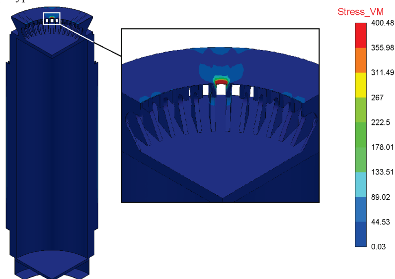
Рисунок 4 – Интенсивность напряжений по Мизесу \sigma_i , МПа
