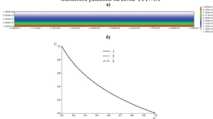
Рисунок 2 – Осесимметричная задача о течении Куэтта: а) Поле скорости u ; б) График сходимости численного решения к аналитическому: 1 – аналитическое решение:
