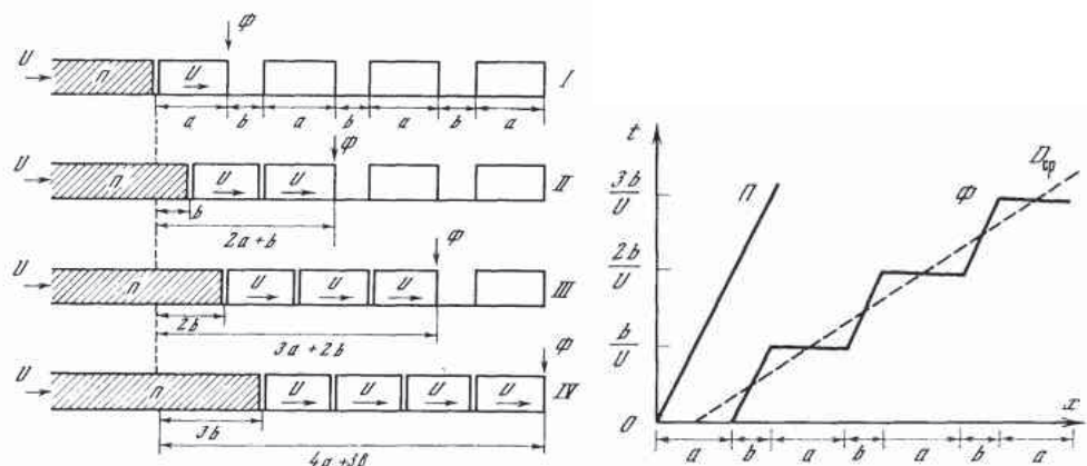
Рисунок 1 – Модель сжатия твердого тела. График фронта ударной волны. x – расстояние, t – время, пунктиром указано усредненное движение фронта
