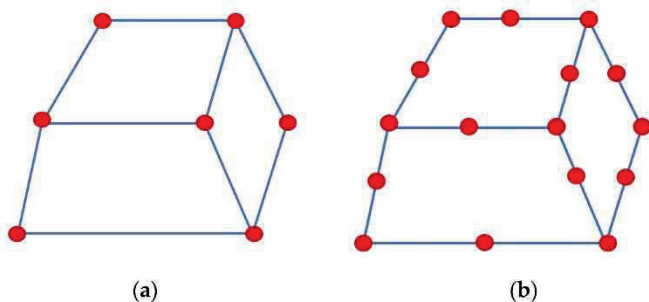
Рис. 2 – Пример разбиения конструкции на конечные элементы
