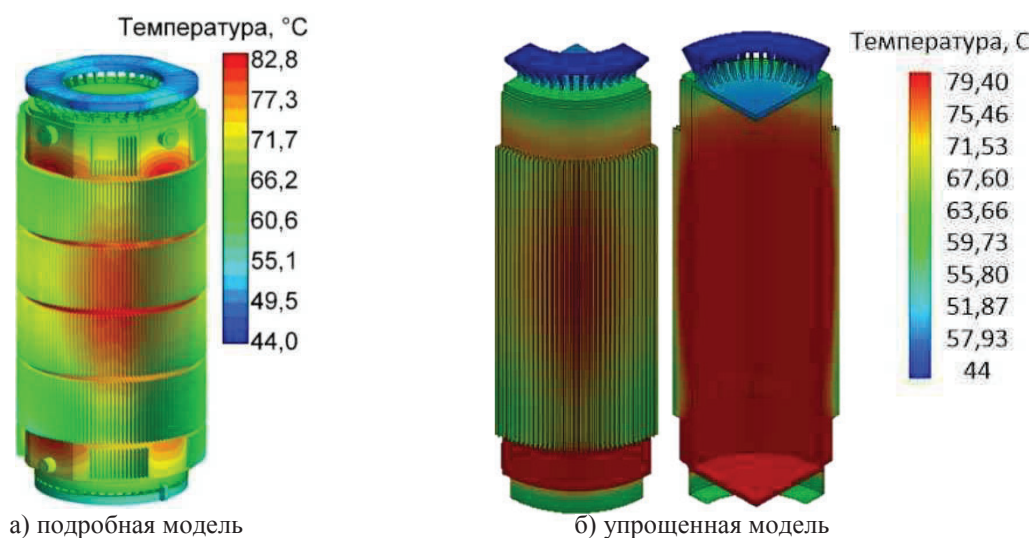
Рисунок 2 – Распределение температур по наружной поверхности ТУК
