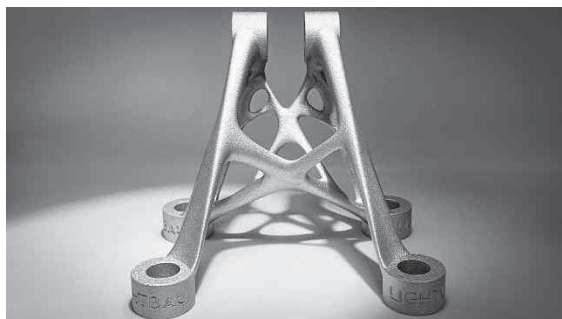
Рис. 4 – Изготовление оптимизированной конструкции с помощью 3D-печати
