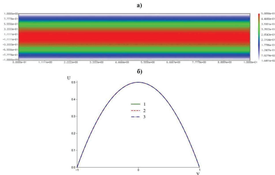
Рисунок 3 – Осесимметричная задача о течении Пуазейля: а) Поле скорости u ; б) График сходимости численного решения к аналитическому: 1 – аналитическое решение:
