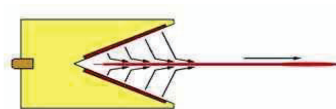
Рис. 1. Кумулятивный поток, образованный в результате столкновения элементов облицовки.
