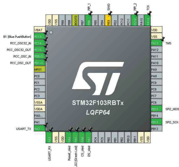
Рис.2. Схема подключения электронных компонентов к контактам платы
