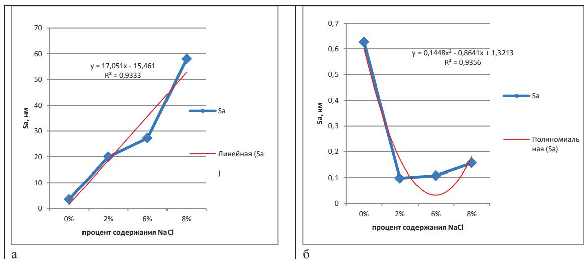
Рис.3- Зависимость шероховатости пленки от концентрации соли: а – скан 30х30мкм; б - для скана 0.1х0.1мкм.
