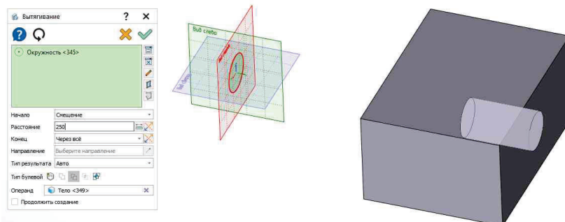
Рис. 6. Вытягивание со смещением, равным 250 и режим конца вытягивания через всё с применением булевой операции вычитания
