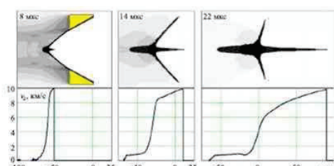
Рис. 2. Формирование кумулятивной струи зарядом с конической облицовкой прогрессивной толщины 1.4...2.6 мм.
