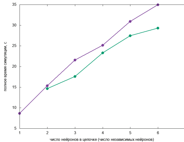
Рисунок 5 - Зависимость полного времени моделирования (total elapsed time) в симуляторе LTspice от параметра «число нейронов». Длительность эпохи симуляции 5кс. Для симуляции использовался компьютер Intel Core i7-3770@3.4GHz 16Gb
