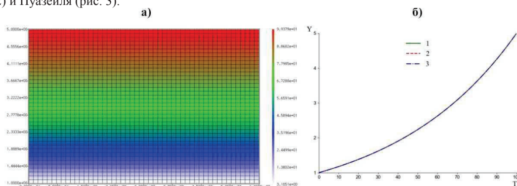
Рисунок 1 – Осесимметричная задача теплопроводности: а) Поле температуры на сетке 51 \times 41 ; б) График сходимости численного решения к аналитическому:
