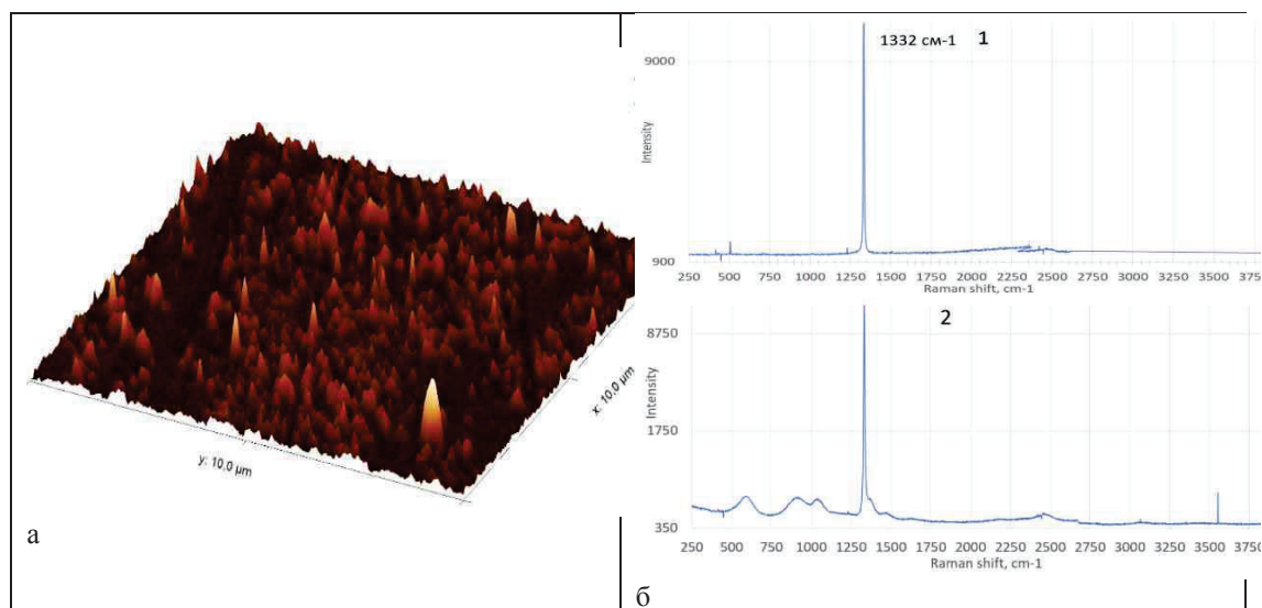
Рисунок 2: а – поверхность образцов CVD-алмаза; б – спектры Рамановской спектроскопии
