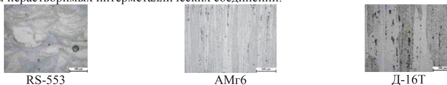
Рисунок 1 – Микроструктура поперечного сечения алюминиевых сплавов
