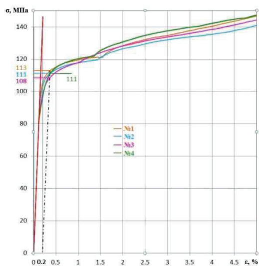
Рисунок 4 – Диаграммы деформирования при сжатии шестикратных образцов из сплава АМцС
