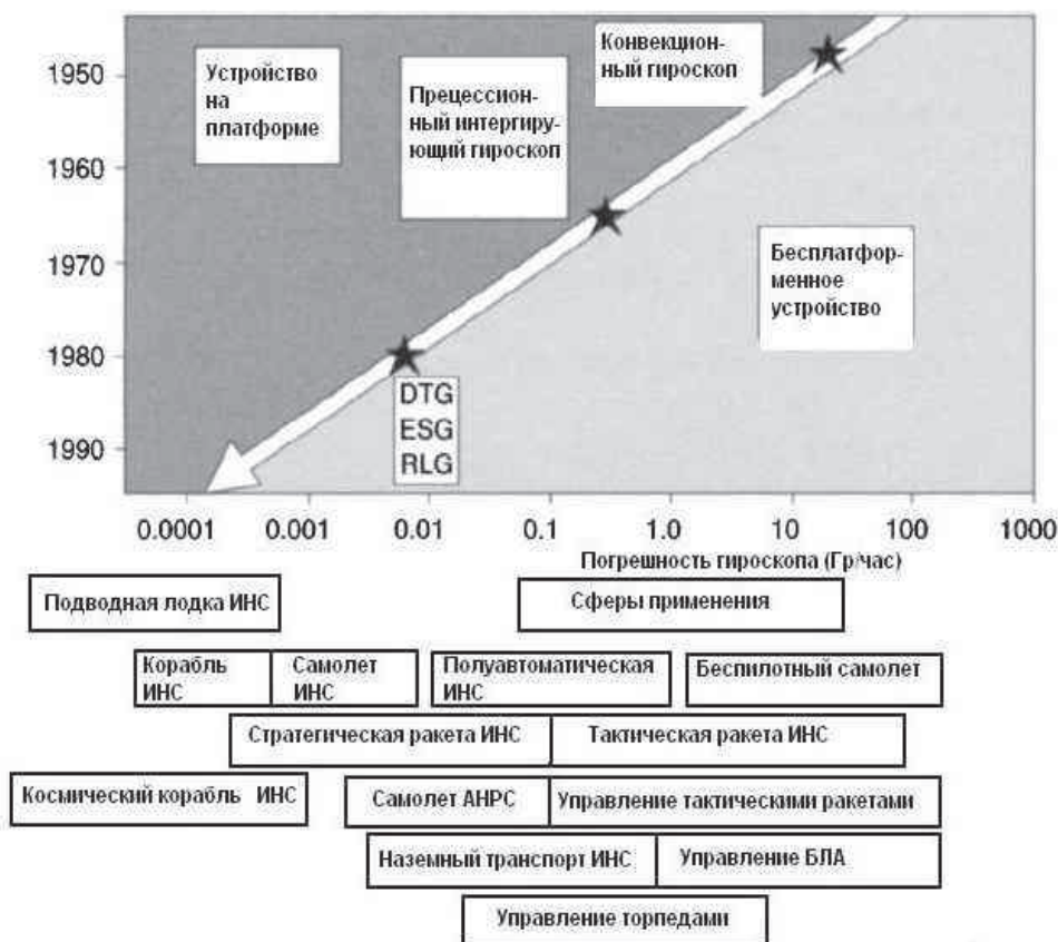
Рисунок 1 – Развитие бесплатформенного датчика и сферы его применения
