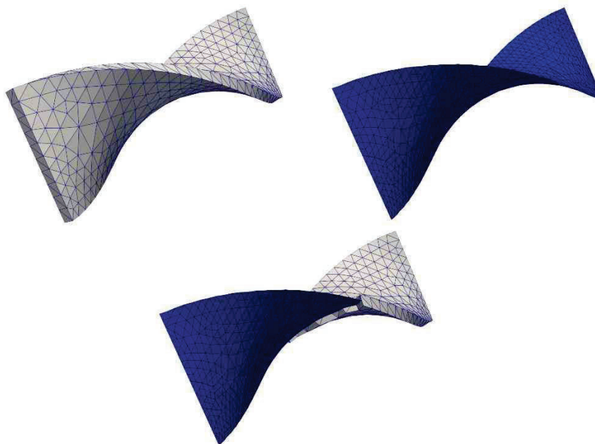
Рис. 2. Срединная поверхность закрученной пластины
