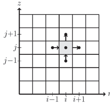
Рис. 2. Расчетная сетка и расположение контрольного объема
