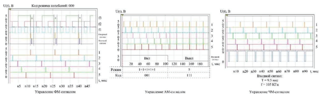
Рисунок 3 – Осциллограммы функционирования моделей систем преобразования
