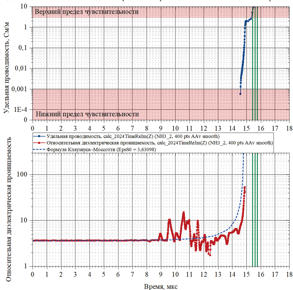
Рис. 3. Графики зависимости удельной проводимости и относительной диэлектрической проницаемости конденсированного аммиака от времени в эксперименте с МК-1. Вертикальные пунктирные линии указывают времена срабатывания бетатронов.
