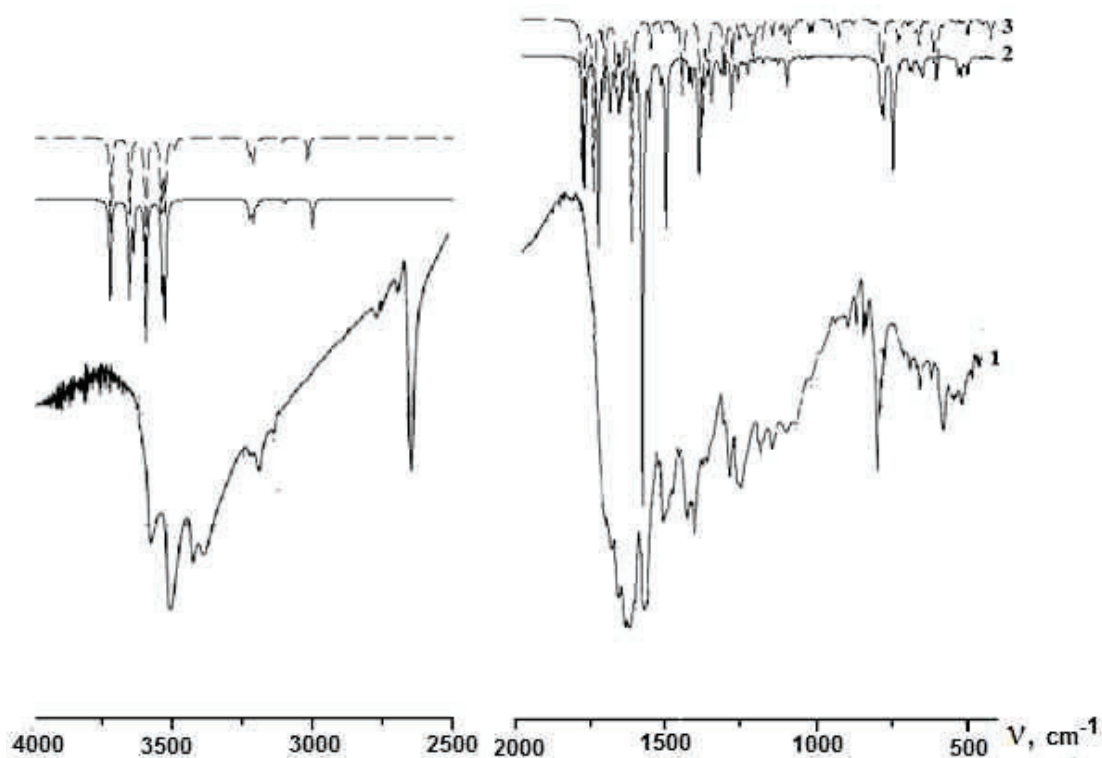
Рис.2. ИК спектры смеси соединений 1a и 1b (эксперимент -1, теория -2, 1a ; 3, 1b )
