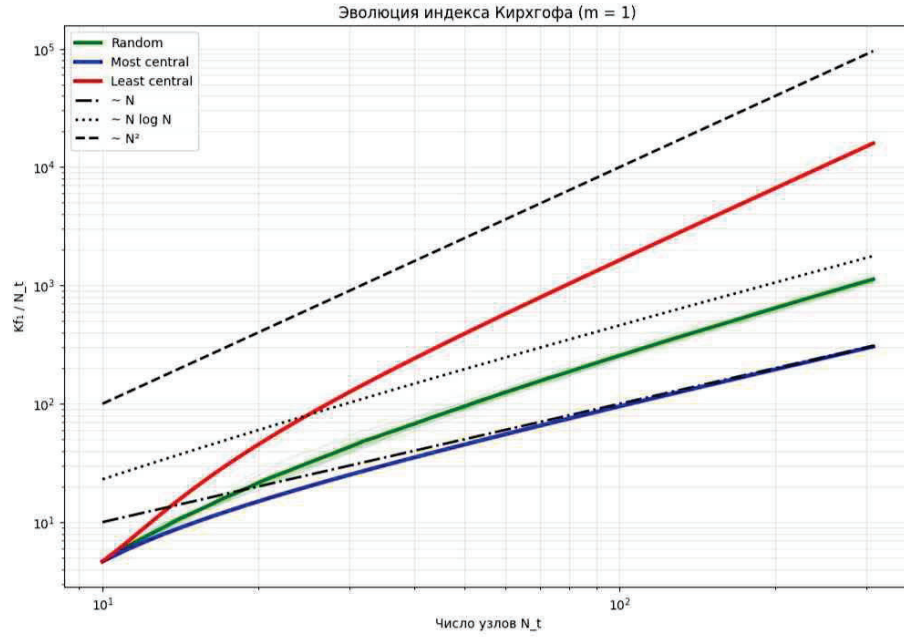
Рис. 1: Эволюция K f / N для m = 1 : зелёный — случайный, синий — наиболее центральный, красный — наименее центральный. Пунктирные линии — теоретические масштабы.
