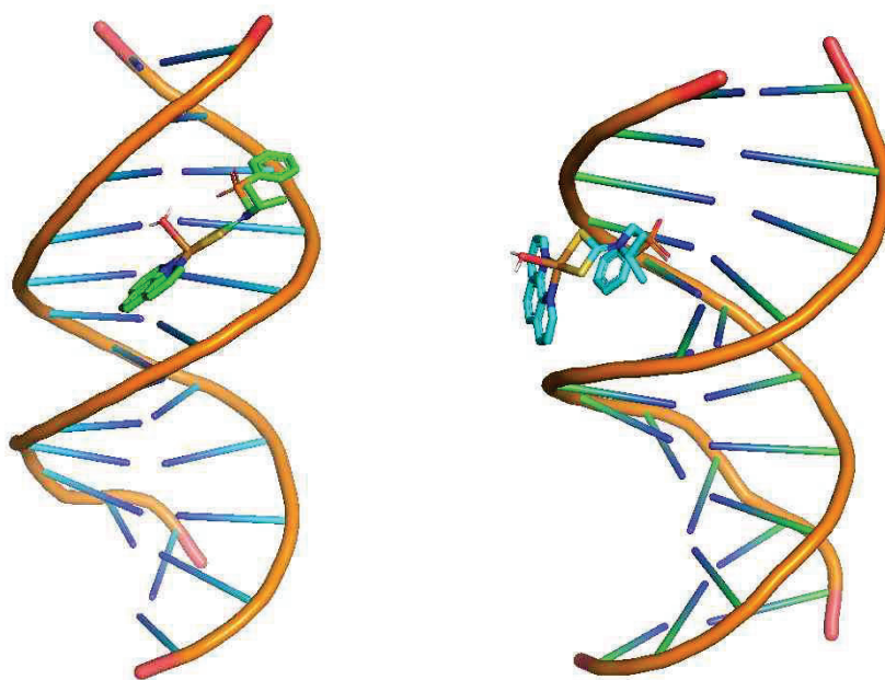
Рис. 3. Расположение комплексов 3 и 3' в молекуле ДНК по данным молекулярного докинга.
