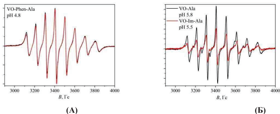
Рис. 2. Экспериментальный и смоделированный спектры ЭПР в системах оксованадий(IV) – 1,10-фенантролин – D - \alpha -аланин; c_{\text{VO(II)}} = 5.00 \cdot 10^{-3} М, c_{\text{Phen}} = 1.023 \cdot 10^{-2} М, c_{\text{Ala}} = 1.249 \cdot 10^{-1} М (А); оксованадий(IV) – D - \alpha -аланин и оксованадий(IV) – имидазол – D - \alpha -аланин; c_{\text{VO(II)}} = 5.00 \cdot 10^{-3} М, c_{\text{Im}} = 1.020 \cdot 10^{-2} М, c_{\text{Ala}} = 2.506 \cdot 10^{-1} М и 1.251 \cdot 10^{-1} М соответственно (Б); T = 25 °С, 1.0 М \text{KNO}_3 .
