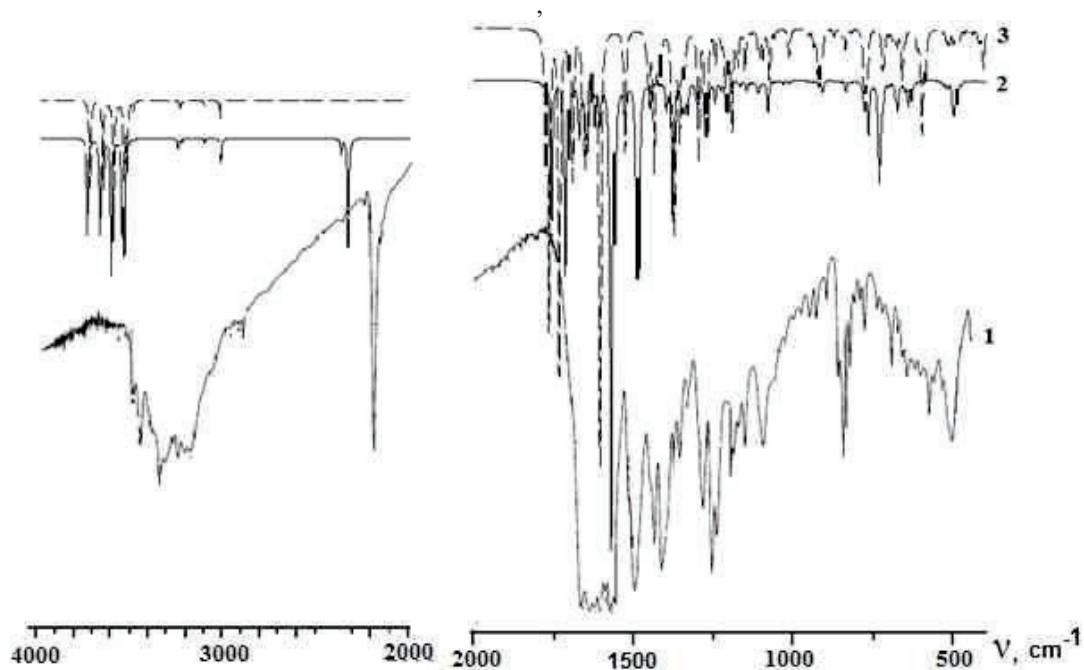
Рис.3. ИК спектры смеси соединений 2a и 2b (эксперимент -1, теория -2, 2a ; 3, 2b ),
