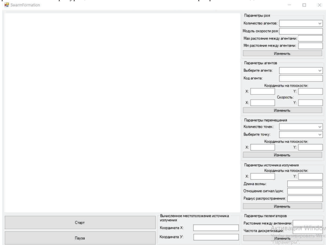
Рисунок 1. Интерфейс программы
