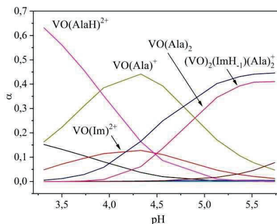
Рис. 3. Диаграмма распределения комплексных форм в системе оксованадий(IV) – имидазол – D -α-аланин в условиях СФ-титрования; c_{\text{VO(IV)}} = 5.00 \cdot 10^{-3} \text{ M} , c_{\text{Im}} = 1.012 \cdot 10^{-2} \text{ M} , c_{\text{D-Ala}} = 2.521 \cdot 10^{-1} \text{ M} ; T = 25 \text{ }^\circ\text{C} , 1.0 \text{ M KNO}_3 .
