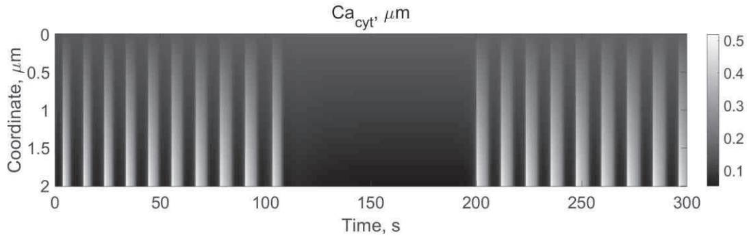
Рис. 2. Пространственно-временное распределение Ca^{2+} в цитозоле, полученное в результате моделирования; типичный результат.
