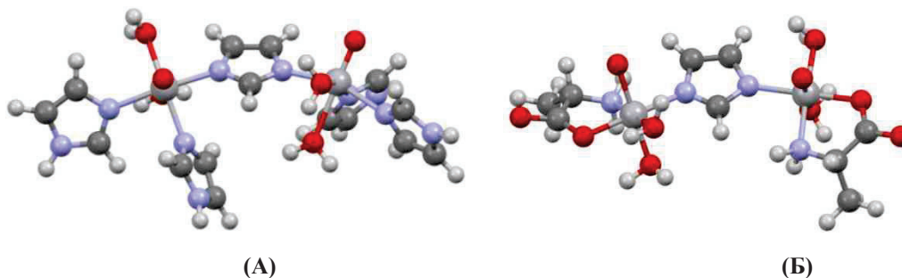
Рис. 1. Структура комплексов (\text{VO})_2(\text{ImH}_{-1})(\text{Im})_4^{3+} (А) и (\text{VO})_2(\text{ImH}_{-1})(\text{Ala})_2^{+} (Б), оптимизированная по программе ORCA [4] методом DFT на уровне B3LYP/def2-TZVPP с коррекцией дисперсии D3 и учетом эффектов растворителя в модели C-PCM.
