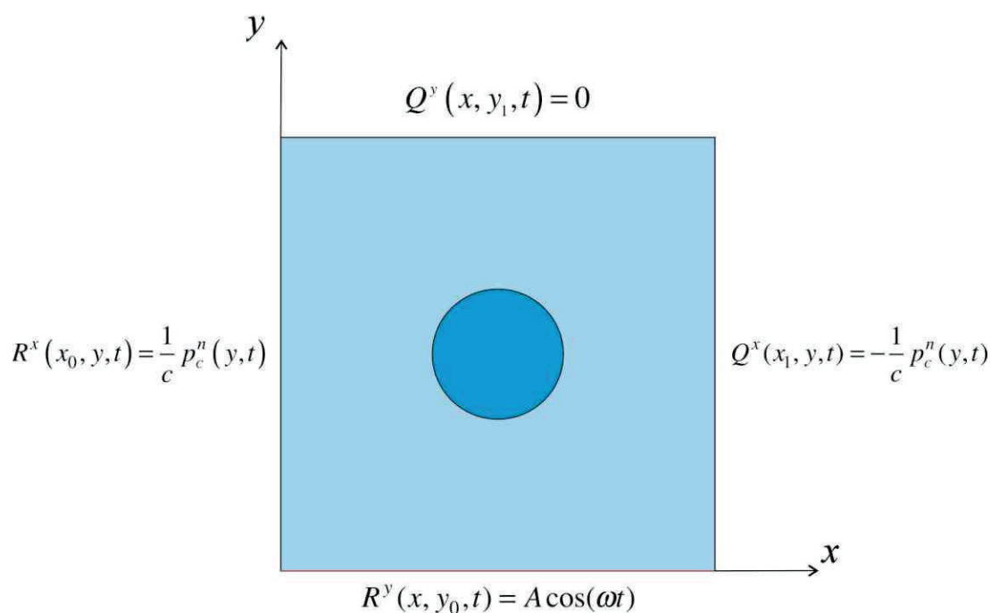
Рисунок 1 – Математическая постановка задачи о рассеянии плоской акустической волны на твёрдом цилиндре с помощью схемы КАБАРЕ
