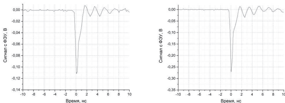
Рисунок 3 - Форма импульсов сигнала с ФЭУ для систем вода-воздух и формамид-воздух
