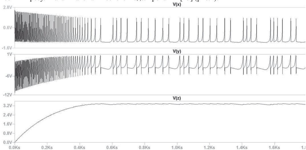
Рисунок 4 - Результаты численного моделирования (симуляции) поведения идеализированной модели РХ-нейрона при помощи симулятора LTspice
