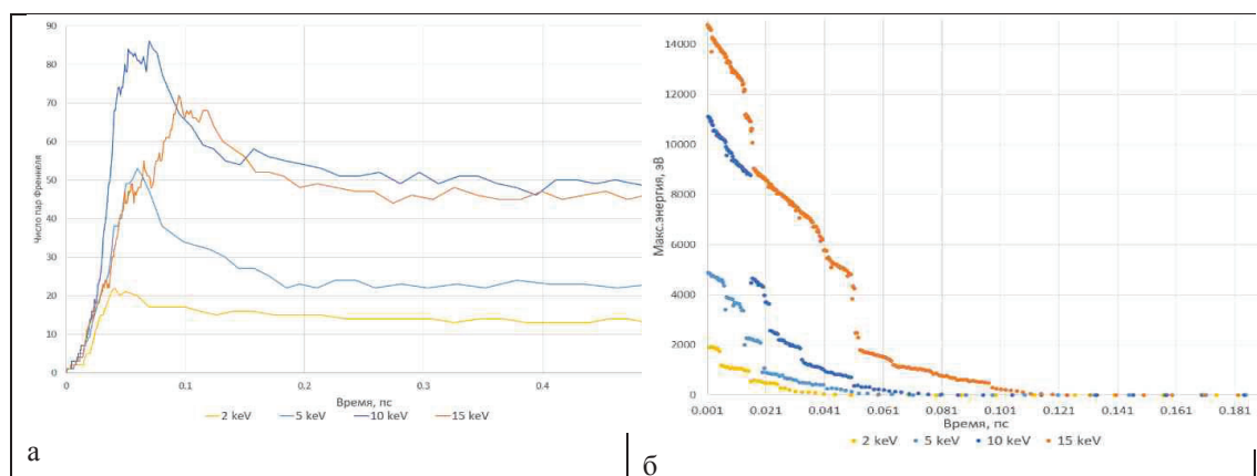
Рисунок 3: а – зависимость числа образованных пар Френкеля от времени процесса; б – зависимость максимальной энергии от времени
